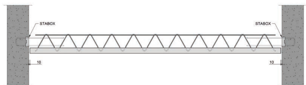
Opleg dragende richting in doorlopende wand
