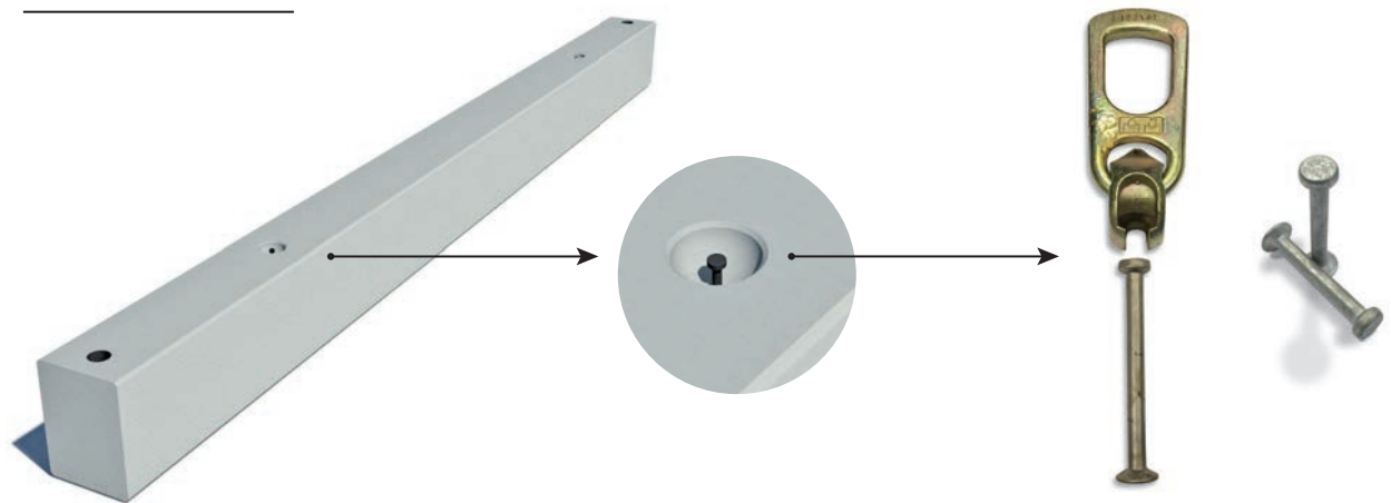
Balk met kogelkopanker
