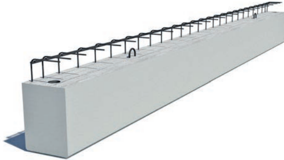
Balk met uitstekende wapening bovenaan
