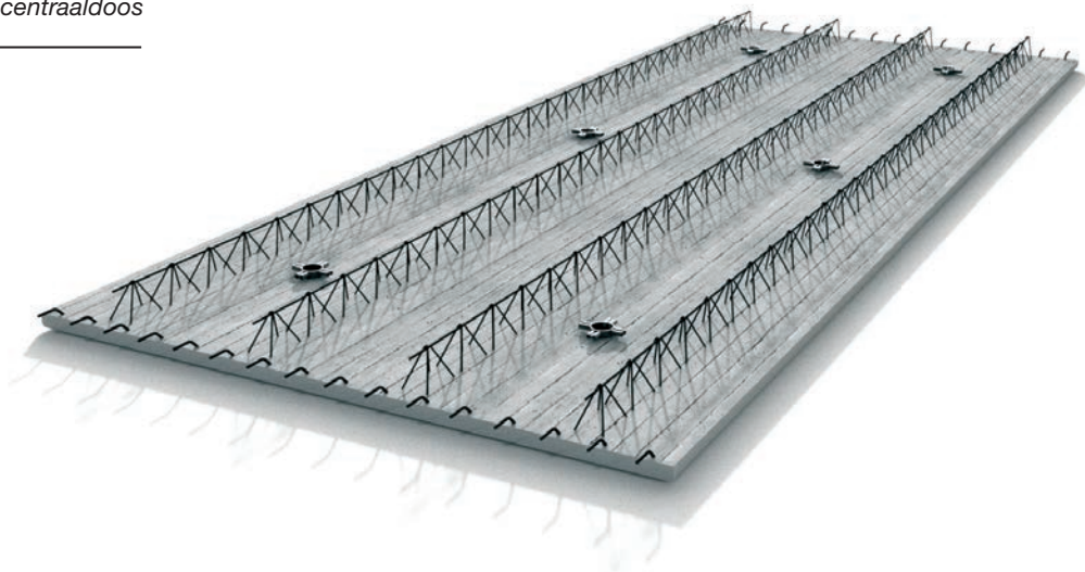
Pedal, 5 cm dik - met centraaldoos
