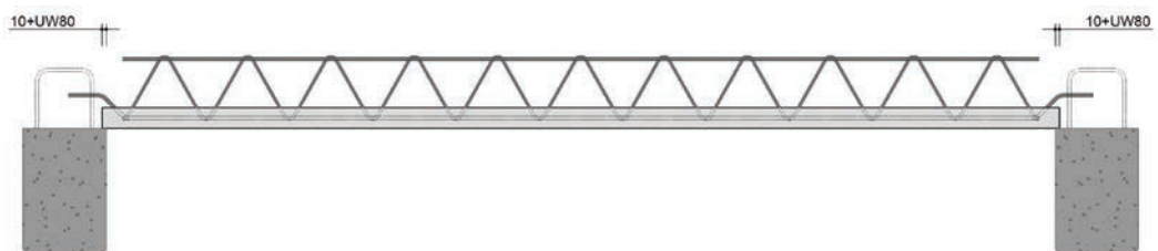
Opleg dragende richting in balk
