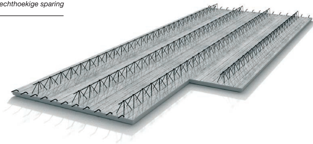
Predal, 5 cm dik - met rechthoekige sparing
