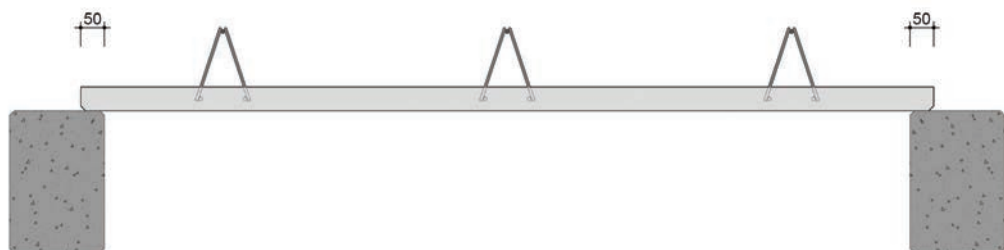
Opleg niet-dragende richting in balk
